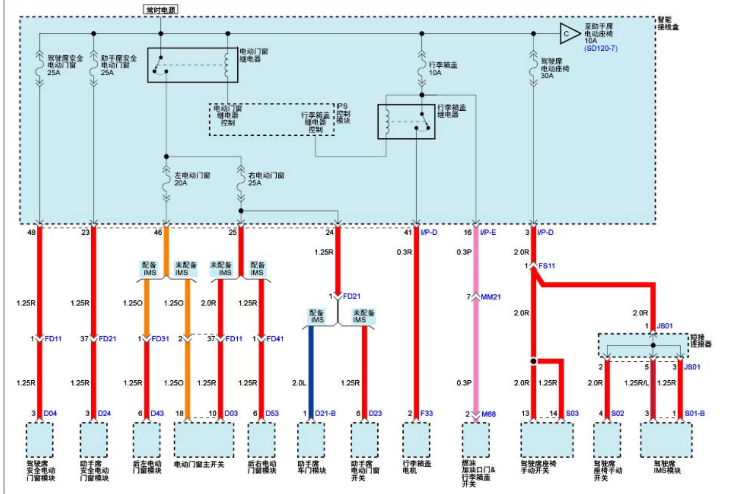
室内保险丝分布(6)
